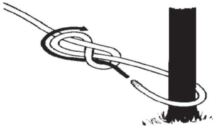
Figure 10B-5 Nœud en huit double
